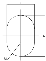
E部詳細
