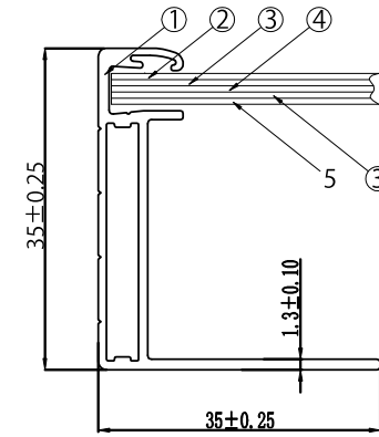
A-A'断面
