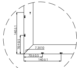
B部拡大
